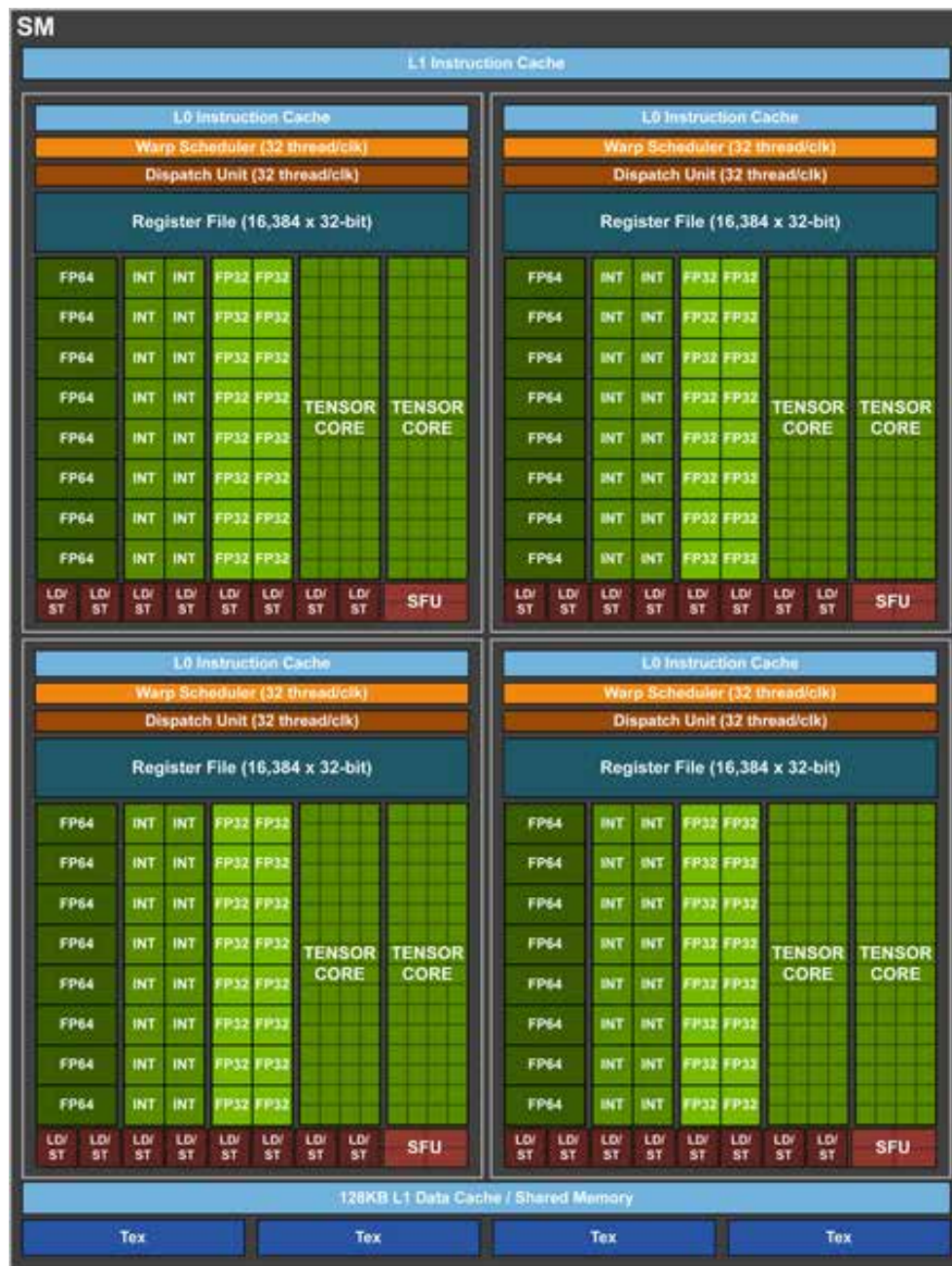
Рис. 5. Архитектура нового мультипроцессора семейства Volta GV100
