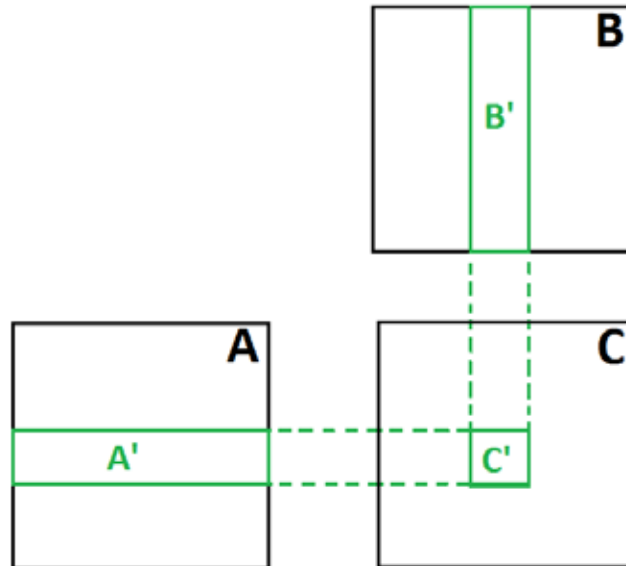
Рис. 7. Вычисление подматрицы новой матрицы
