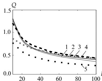
Рис. 10. Численный расчет и приближенные оценки дебита ГС: 1 – численный расчет, 2 – приближенный расчет, 3 – формула Борисова, 4 – формула Гигера–Райса, 5 – формула Джоши
