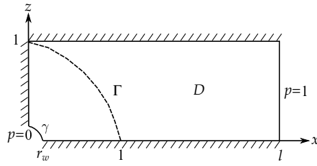
Рис. 6. Область решения задачи о притоке жидкости к горизонтальной скважине
