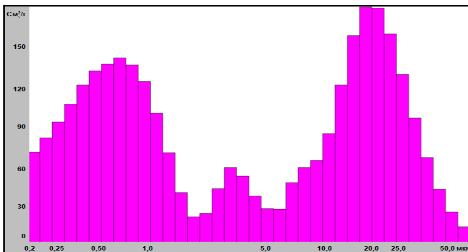
Рисунок 2 – Гистограмма удельной поверхности частиц ( \text{см}^2/\text{г} ) \text{Al}_2\text{O}_3
