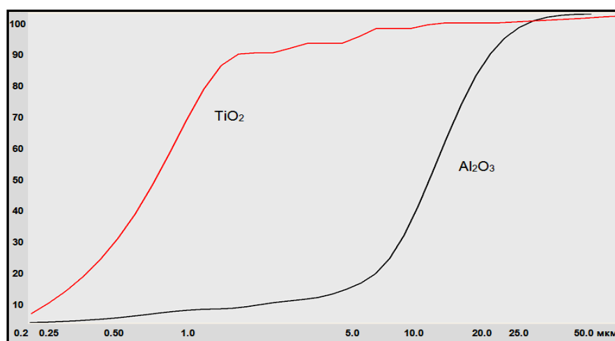
Рисунок 1 – Интегральное распределение (P,%) весовых долей частиц Al 2 O 3 и TiO 2
