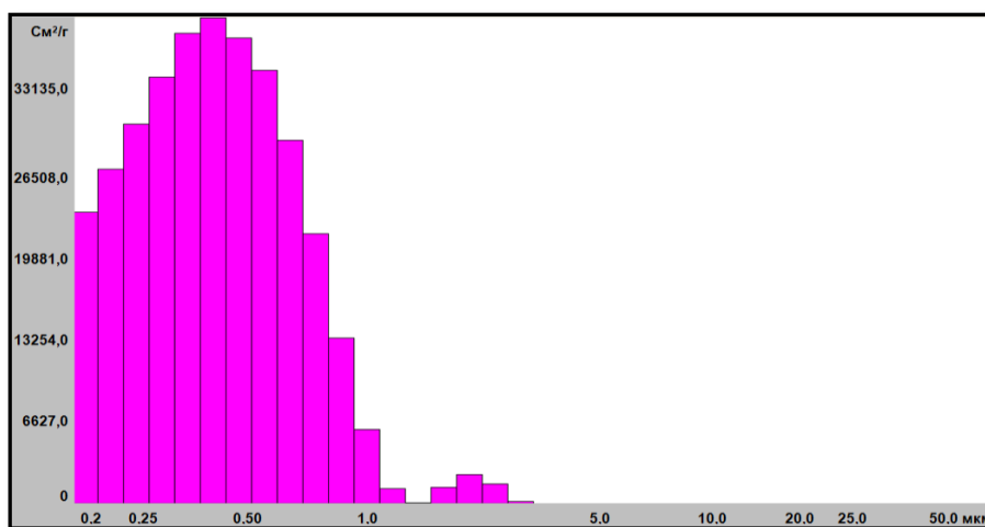
Рисунок 3 – Гистограмма удельной поверхности частиц ( \text{см}^2/\text{г} ) \text{TiO}_2
