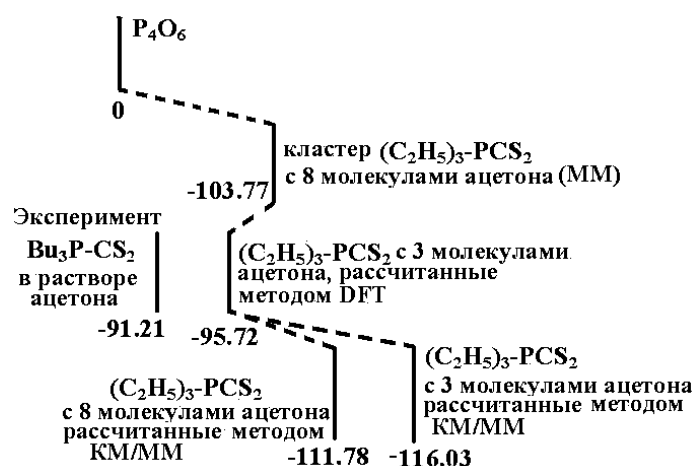
Рис. 4. Диаграмма относительных изменений химических сдвигов ядра ^{31}\text{P} молекулы (\text{C}_2\text{H}_5)_3\text{P-CS}_2 в кластерах с разным числом молекул ацетона, рассчитанных различными методами, в сравнении с экспериментальным значением для \text{Bu}_3\text{P-CS}_2 в растворе ацетона
