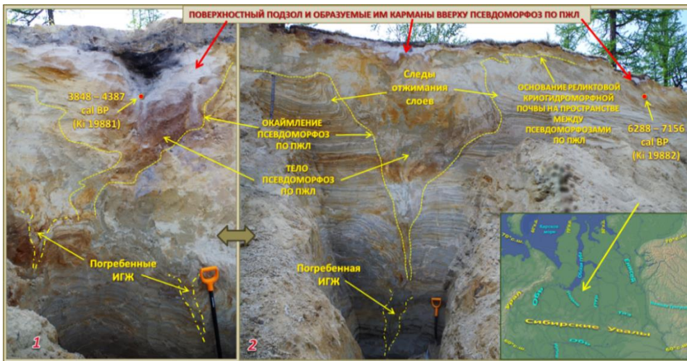
Рисунок 1. Расчистка стенки карьера в верхьях р. Правая Хетта. Фото В.С. Шейнкмана. Сокращения: ПЖЛ – полигонально-жильный лед; ИГЖ – изначально-грунтовая жила.
