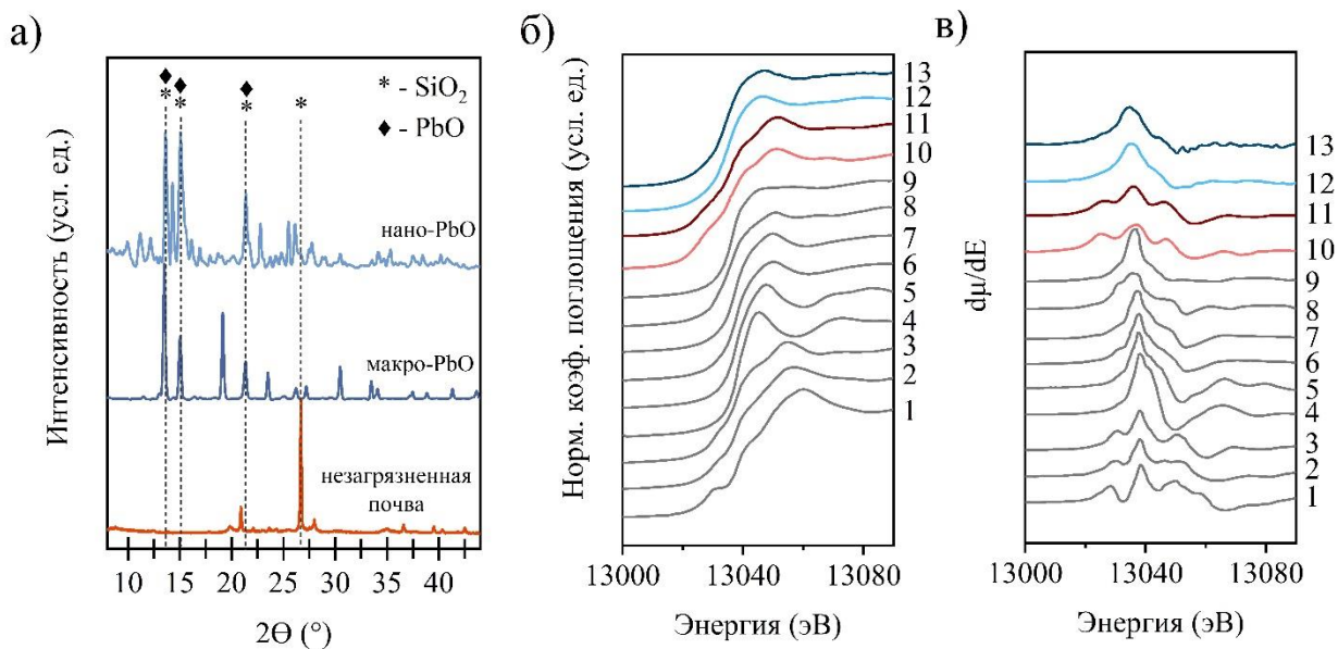
Рисунок 1. Дифрактограммы озоленных корней ячменя ярового, загрязненных нано- (12) и макроформами (13) \text{Pb} и незагрязненной почвы (а), а также спектры рентгеновского поглощения (б) и их первые производные (в) в сравнении с эталонами: \text{PbO}_2 (1), \text{Pb}_3\text{O}_4 (2), \text{PbO} (3), \text{Pb}(\text{NO}_3)_2 (4), \text{PbCO}_3 (5), \text{Pb}(\text{CH}_3\text{COO})_2 (6), \text{Pb}(\text{CH}_3\text{COO})_2 \cdot 3\text{H}_2\text{O} (7), \text{PbS} (8), \text{PbCl}_2 (9), нано- \text{PbO} (10), макро- \text{PbO} (11)
