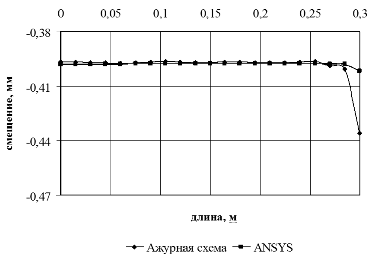
Рис. 7. Сравнение решений
