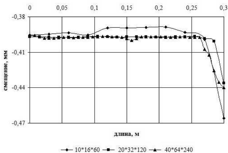
Рис. 6. Сходимость решения
