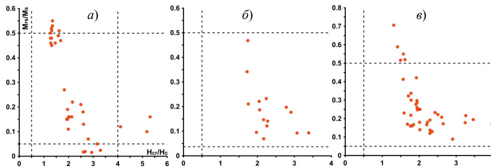
Рис. 5. Диаграммы Дзя: M_{Ts}/M_s по отношению к H_{cr}/H_c : а – разрез Ергалах; б –дельканская свита; в – тыванкитская свита
