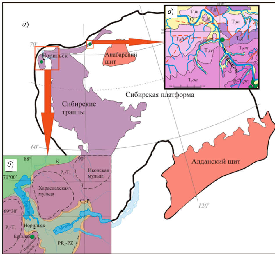
Рис. 1. а – местоположение изученных разрезов на Сибирской платформе; б – геологическая схема Норильского района; в – геологическая схема района р. Маймечи. P 2 -T 1 gr – правобоярская свита; T 1 on – онкучакская свита; T 1 tv – тыванкитская свита; T 1 dl – дельканская свита; T 1 m – маймечинская свита; T 1 g – дуниты Гулинского массива
