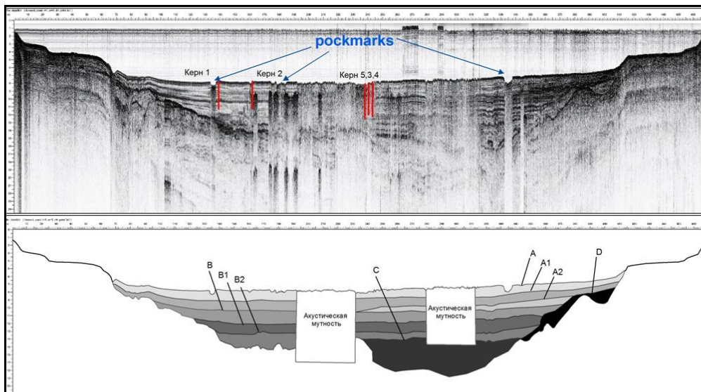
Рис. 2. Сейсмоакустический разрез 2. Отображение разреза с детектированием сигнала. На разрезе отмечены места отбора керновых колонок. Стрелками указаны покмарки (верхний рисунок). Предварительный сеймостратиграфический анализ (нижний рисунок) позволяет выделить 8 границ – этапов формирования донных отложений (А, А1, А2, В, В1, В2, С, D)
