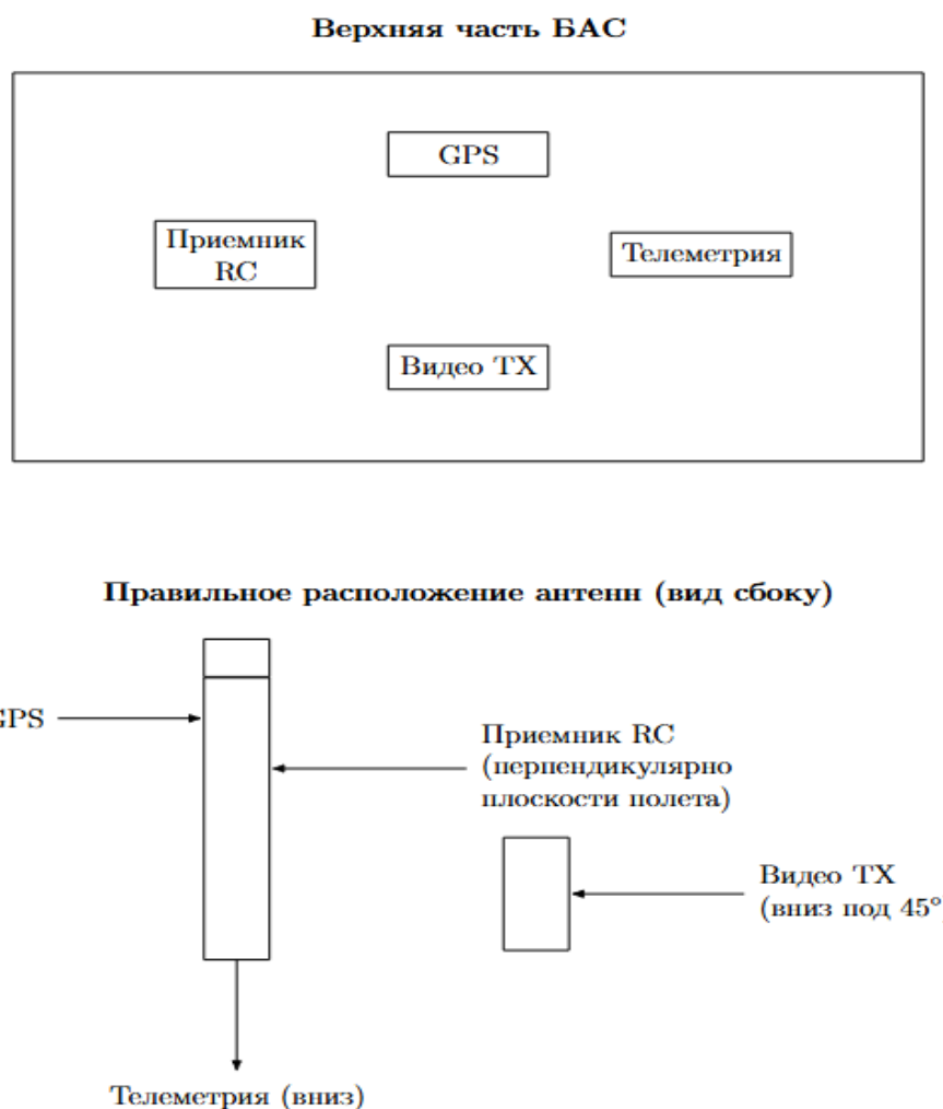
Рис. 18. Типовая схема расположения антенн на БАС
