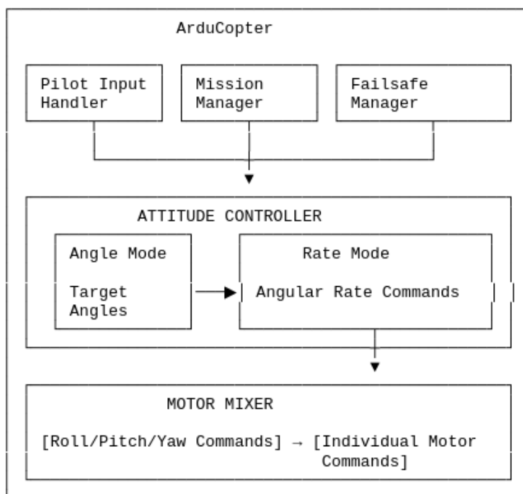
Рис. 79. Структура ArduCopter
