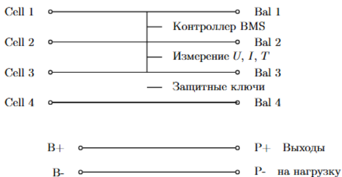
Рис. 40. Схема BMS для многоэлементной батареи
