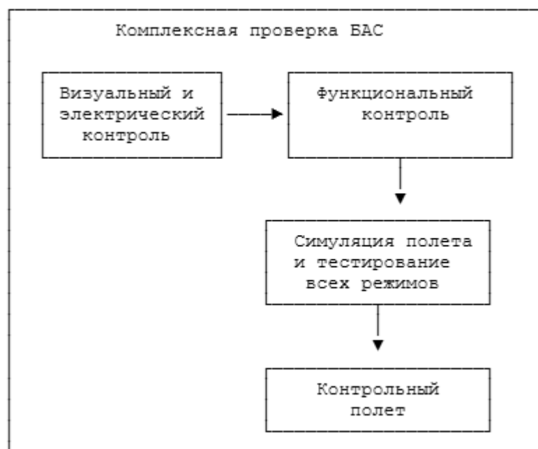
Рис. 16. Схема проверки электронных компонентов после восстановления
