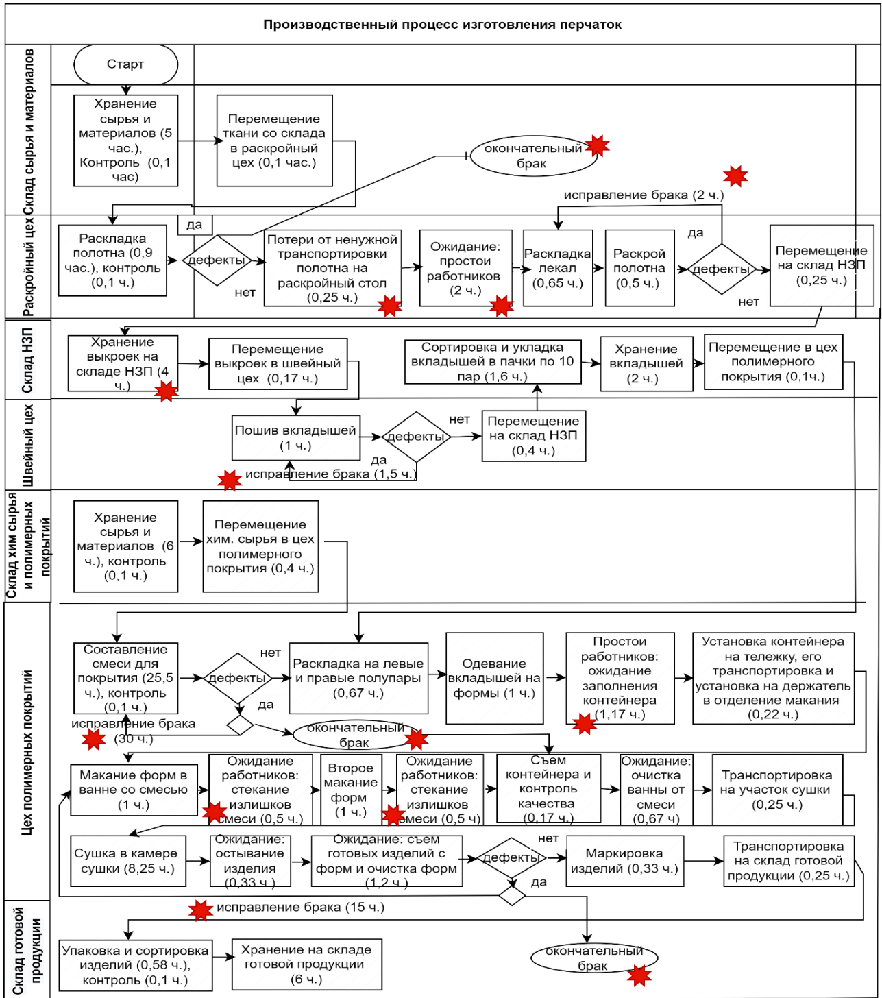
Рис. 1. Карта процесса изготовления перчаток
