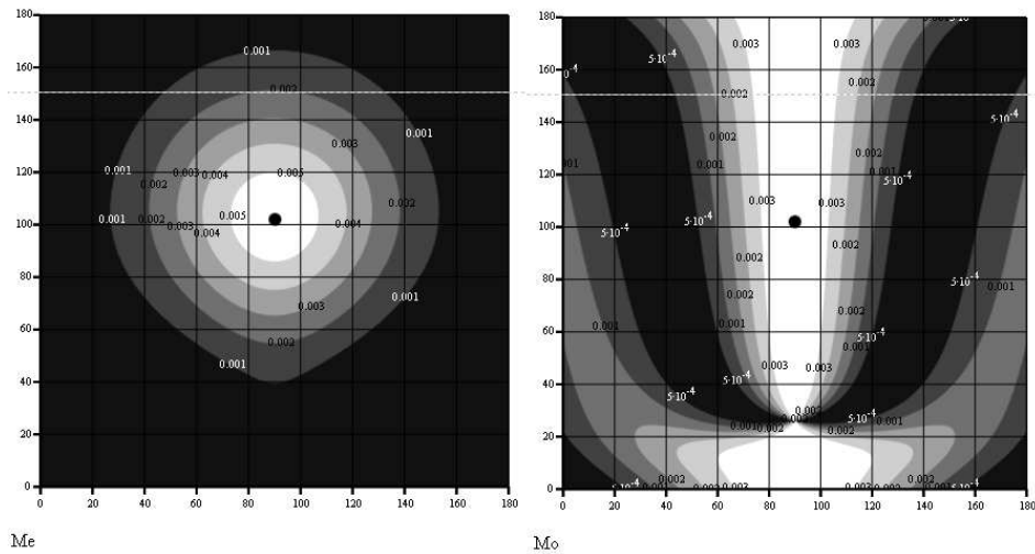
Рис. 1. Пространственное распределение акустооптического качества для e -волны (слева) и o -волны (справа). Направление света для оптимального среза указано точкой
