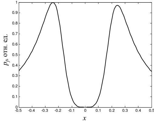
Рис. 3. Зависимость вероятности двухфотонного поглощения p_f от расстройки x = \Delta/\omega_{fg} при z/z' = 10^{-2}
