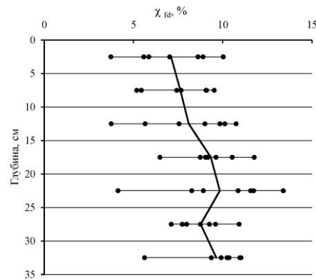
Рис. 6. Частотно-зависимая магнитная восприимчивость образцов из верхней части профилей залежной светло-серой лесной почвы как функция от глубины
