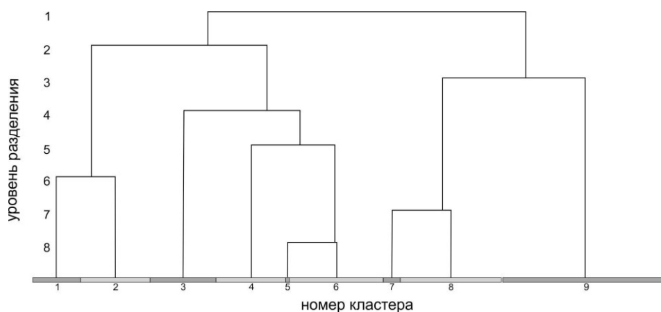
Рис. 2. Дендрограмма полученная при обработке геоботанических описаний методом модифицированного TWINSPLAN. Длина отрезка по оси абсцисс отражает количество описаний, вошедших в данный кластер
