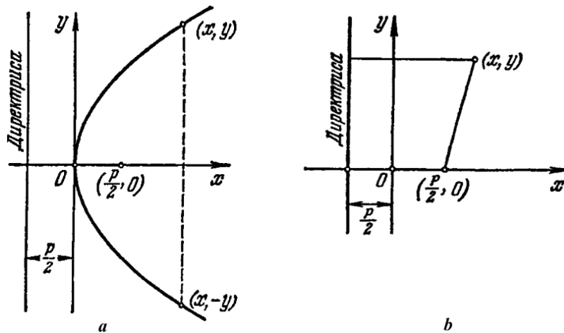
Рис. 4. К описанию геометрических свойств параболы (a). К определению параболы (b)
