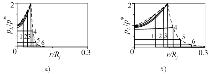
Рис. 2. Радиальные профили нагрузки (1) для шести моментов времени при v_j = 100 м/с (а) и v_j = 300 м/с (б)
