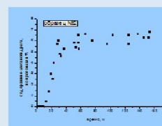
Рис.8. Зависимость процентного содержания гидрата от времени во втором образце, в стандартных условиях (T=7°C, p=100атм)
