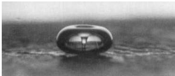
Рис. 3. Фотография пузырька, схлопывающегося у стенки с образованием на его поверхности высокоскоростной струи [6]
