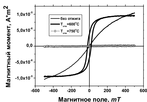
Рис. 4. Зависимости магнитного момента нанокompозитной пленки \text{Co:BaTiO}_3 от магнитного поля для различных температур отжига пленки
