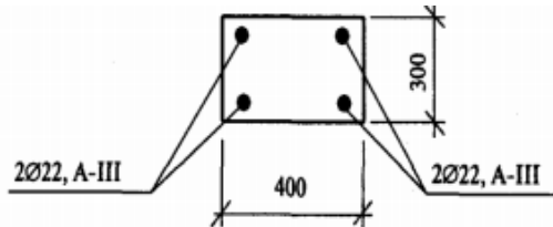
Рис1 Сечение колонны.
