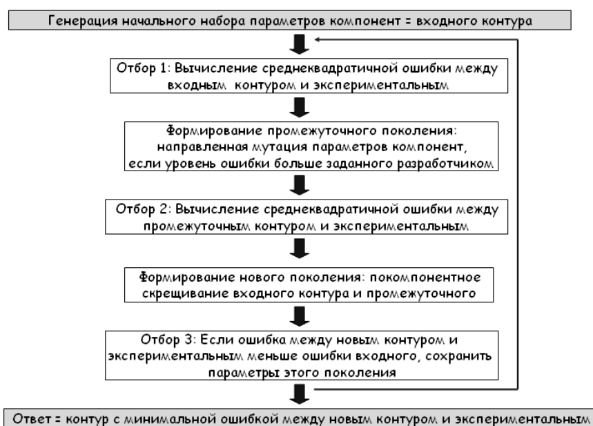
Рис. 2. Генетический алгоритм для обработки спектральных данных
