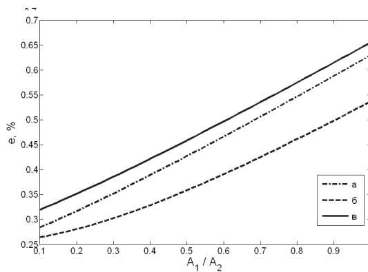
Рис. 6. Зависимость среднеквадратичной ошибки ( e ) восстановления суммарного контура от отношения интенсивностей полос A_1/A_2 : а) полуширина 12\text{ см}^{-1} , расстояние между полосами 1.75\text{ см}^{-1} ; б) полуширина 12\text{ см}^{-1} , расстояние между полосами 2.5\text{ см}^{-1} ; в) полуширина 14\text{ см}^{-1} , расстояние между полосами 2.25\text{ см}^{-1}
