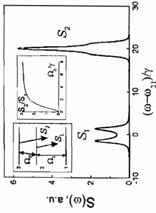
Рис. 2. Спектр резонансной флуоресценции мессбауровского излучения, \gamma = 1 , \Omega_0 = 1.5\gamma , \Omega_1 = 0.01\gamma , D = 0.5\gamma . На вставках схема уровней и зависимость отношения интенсивностей упругого и рамановского каналов рассеяния от частоты Раби р.ч. поля.
