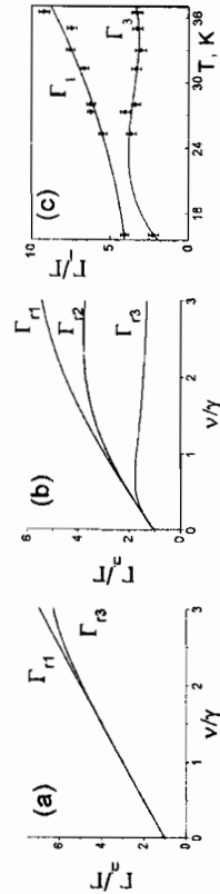
Рис. 10. Расчетные значения релаксационных ширины \Gamma_\gamma линий (см рис. 9). а) v_1 = v_2 = v ; б) v_1 = v , v_2 = 10v ; в) Зависимость ширины линий 1 и 3 от температуры, измеренная экспериментально для \text{FeCO}_3 .
