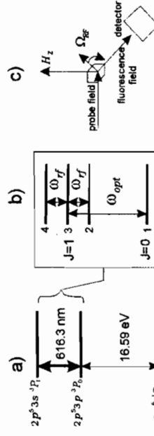
Рис. 6. а) Структура энергетических уровней атома неона. б) Переход 2p^3s^3P_1 \rightarrow 2p^3s^3P_0 . в) Геометрия эксперимента.
