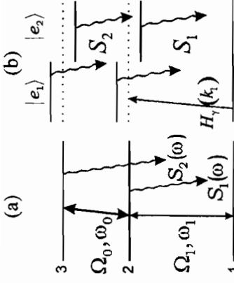
Рис. 1. (а) Трехуровневая мессбауэровская система. \Omega_0 и \Omega_1 – частоты Раби, \omega_0 и \omega_1 несущие частоты управляющего и пробного поля соответственно. (б) Эквивалентная схема в представлении КЭ состояний.
