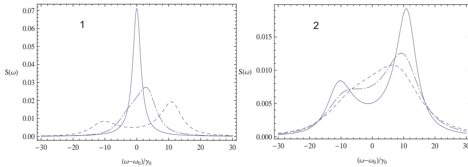
Рис. 1. Контур линии излучения системы двух взаимодействующих атомов: 1) для различных расстояний между атомами: kR = 10\pi (сплошная линия), kR = \pi/6 (штрих-пунктирная линия), kR = \pi/8 (пунктирная линия); 2) для различных температур: N = 1 (сплошная линия), N = 2 (штрих-пунктирная линия), N = 3 (пунктирная линия)
