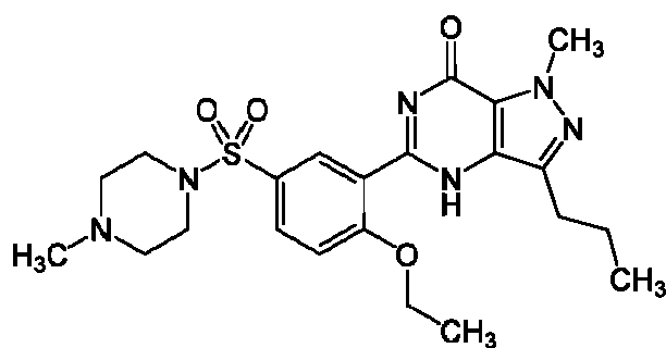
Рис. 1. Структура силденафила
