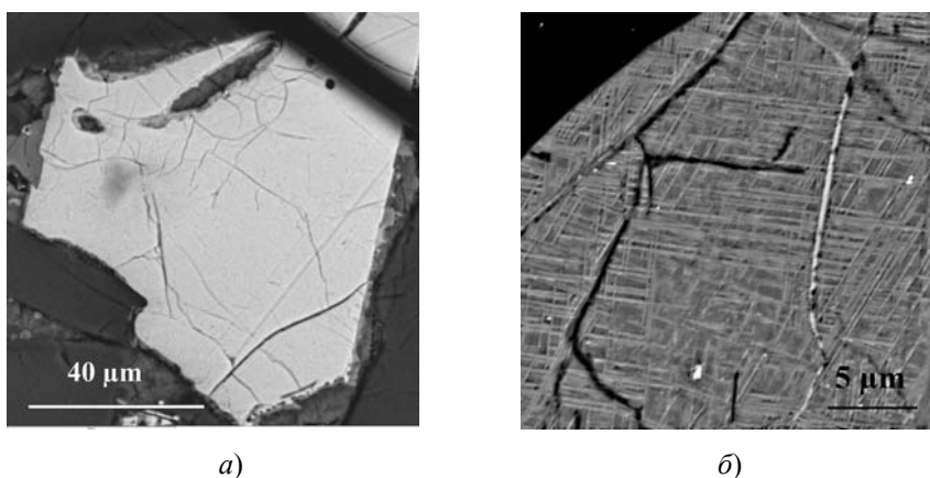
Рис. 1. Микрофотографии (в обратно рассеянных электронах) полированных поверхностей шлифов образца в исходном состоянии ( a ) и термообработанного на воздухе в течение 100 ч при 500 °С ( б ); a – крупное зерно титаномагнетита (светло-серое) первой генерации с мозаичной поверхностью, что является надежным оптическим признаком однофазного окисления, б – тонкие ориентированные ламели ильменита (светлое), образованные в результате гетерофазного окисления титаномагнетита; протравлено HCl
