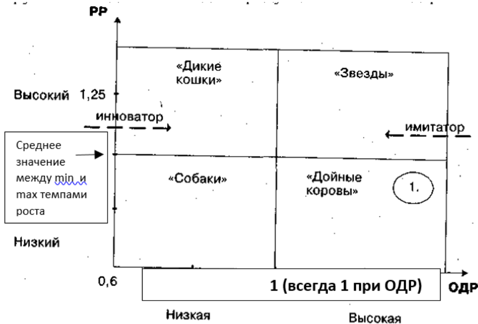
Рис. 1. Матрица БКГ.
