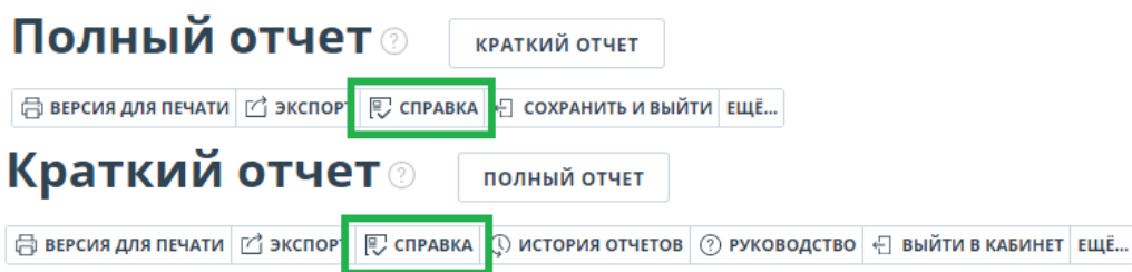
Рисунок 7. Кнопка «Справка».
