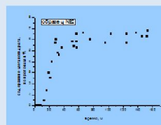
Рис.8. Зависимость процентного содержания гидрата от времени во втором образце, в стативных условиях (T=7С, p=100атм.)
