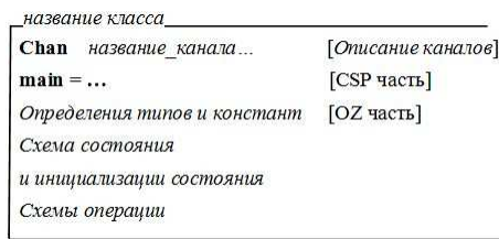
Рис. 3. Основная структура CSP-OZ класса
