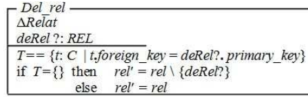
Рис. 17. Схема ограничения операции удаления в Z
