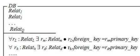
Рис. 11. Схема состояния базы данных в Z
