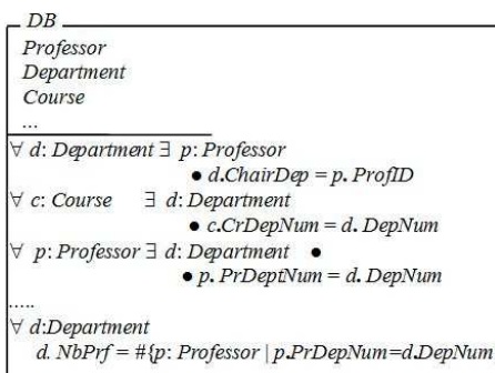
Рис. 12. Схема состояния базы данных «Университет» в Z
