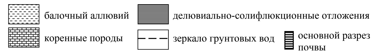
Рисунок 3. Принципиальные схемы расположения основных и поперечных почвенных разрезов в балке в связи с её геолого-геоморфологическим строением (вверху – плановый вид балки, внизу – поперечный разрез балки). 1 – линия профиля ПТК, 2 – основной разрез почвы, 3 – поперечный разрез почвы (полуяма), 4 – направление миграции вещества (талых и дождевых вод, взвешенных, влекаемых и растворённых веществ и т.д.).
