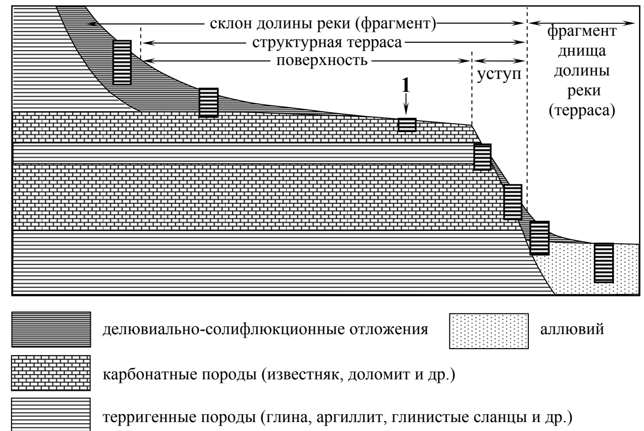
Рисунок 4. Влияние литолого-геоморфологической неоднородности склона долины реки на расположение основных почвенных разрезов; 1– основной разрез почвы.
