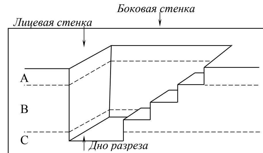
Рисунок 5. Схематичный вид основного почвенного разреза (ямы) А В С – генетические горизонты почвы
