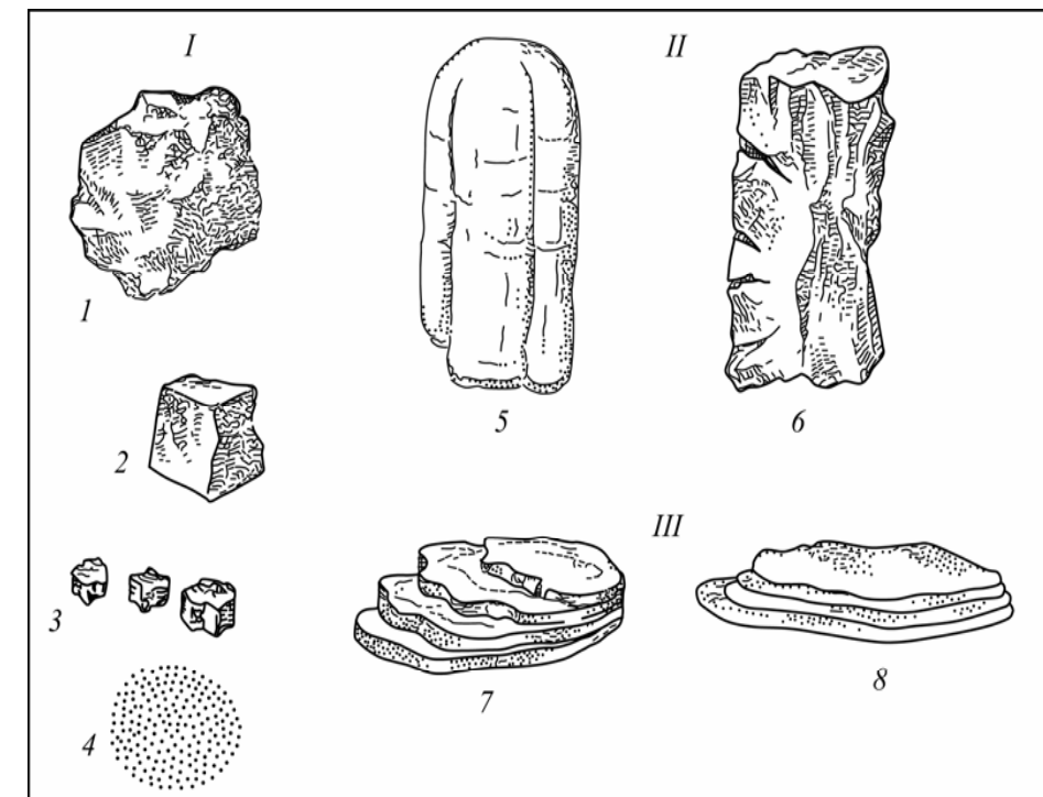
Рисунок 7. Морфология видов структурных элементов (педов): I – кубовидный тип (1 – комковатая структура, 2 – ореховатая, 3 – зернистая, 4 – пылеватая); II – призмовидный тип (5 – столбчатая структура, 6 – призматическая); III – плитовидный тип (7 – пластинчатая структура, 8 – листоватая).
