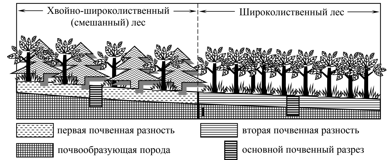
Рисунок 8. Пример установления границы (1) между почвенными разностями сравнительно-генетическим методом В.В. Докучаева по смене растительного покрова.
