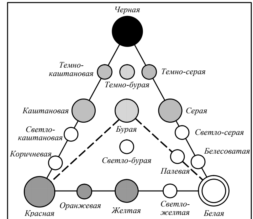
Рисунок 6. Треугольник цветов С.А. Захарова (1931)
