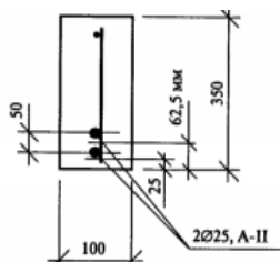
Армирование на рис.1
