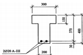
Армирование балки на рис.1
