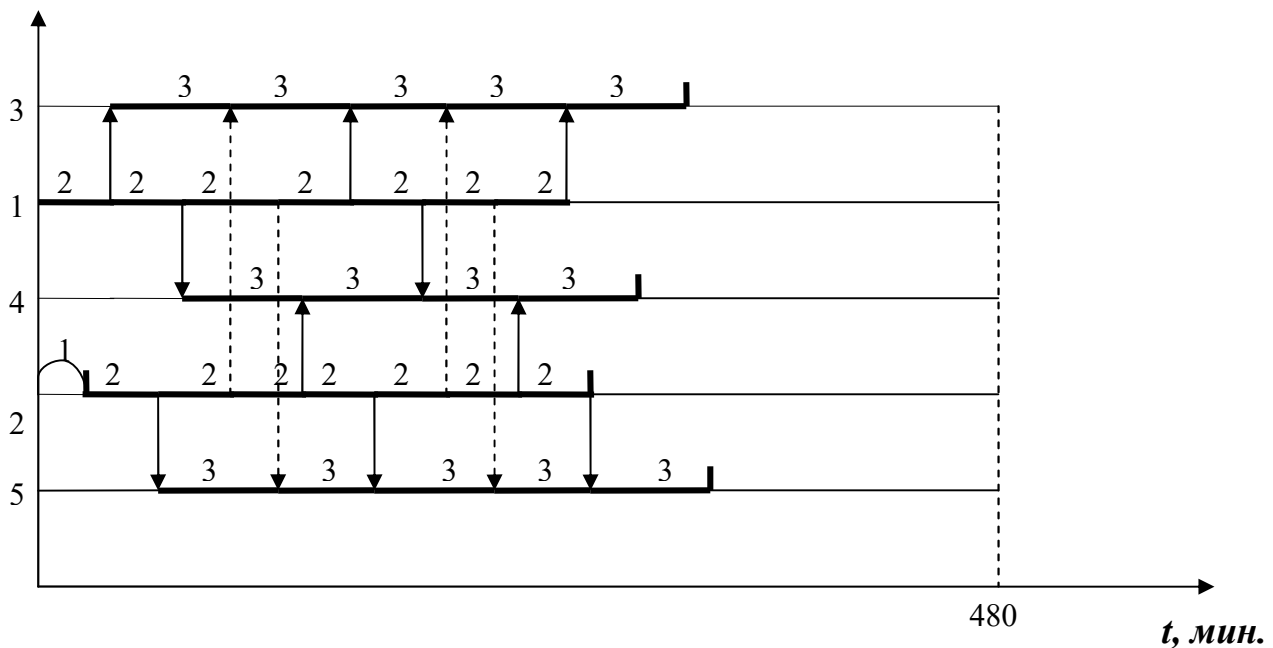
Рис. 3. Ритм работы оборудования на пяти технологических линиях
