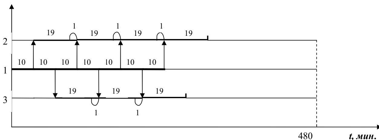
Рис. 2. График работы оборудования на трех технологических линиях
