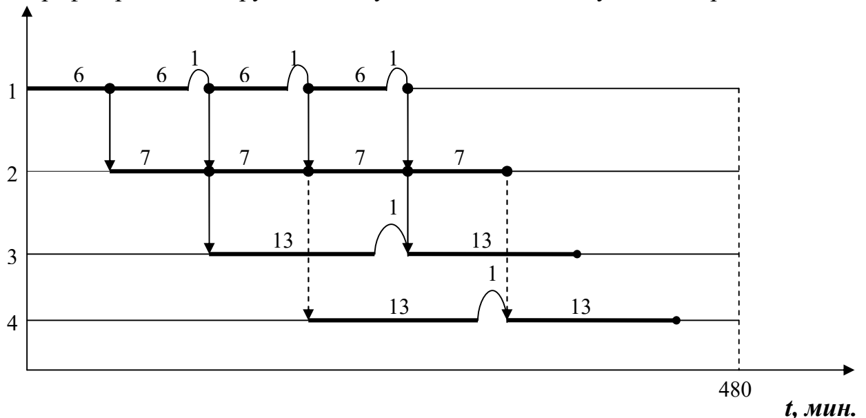
Рис. 4. Ритм работы оборудования на четырех технологических линиях
