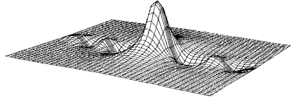
Рис. 1. Общий вид 2D-решений уравнения GKP: \gamma = 1 , \beta = -0,8 ( t = 0,2 ) (а); \gamma = 1 , \beta = 3,16 ( t = 0,5 ) (б)
