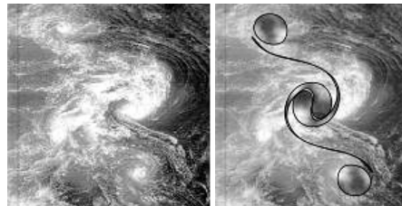
Рис. 4. Моделирование 4-вихревого взаимодействия в канале Naruto (Япония) (справа – численный эксперимент, слева – аэрофотосъемка)
