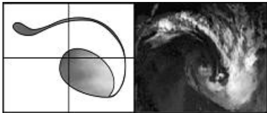
Рис. 3. Моделирование эволюции синоптических вихрей циклонического типа (слева – численный эксперимент, справа – спутниковая фотография)
