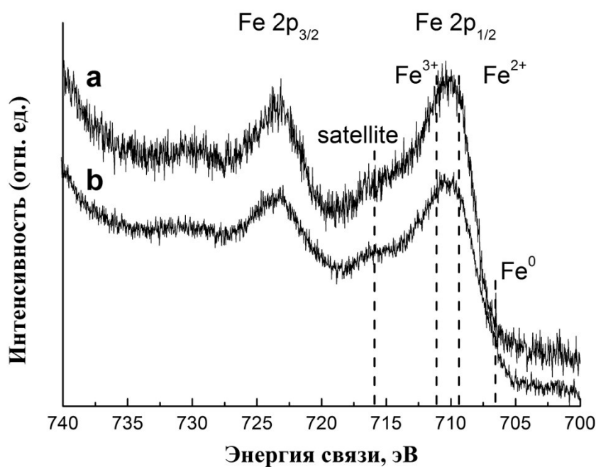
Рисунок 2. ФЭ-линии Fe 2p, записанные на глубине анализа 2-80 нм для пластинки кварца, имплантированной ионами железа с дозой 1 \times 10^{17} ион/см 2
