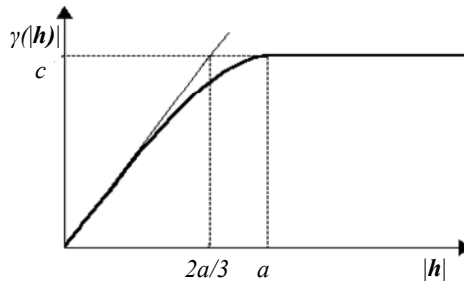
Рис.37. Сферическая модель
