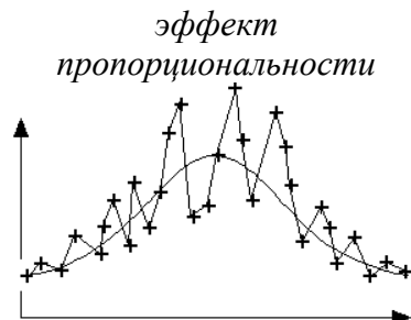
Рис.13. Два примера с непостоянной локальной дисперсией
