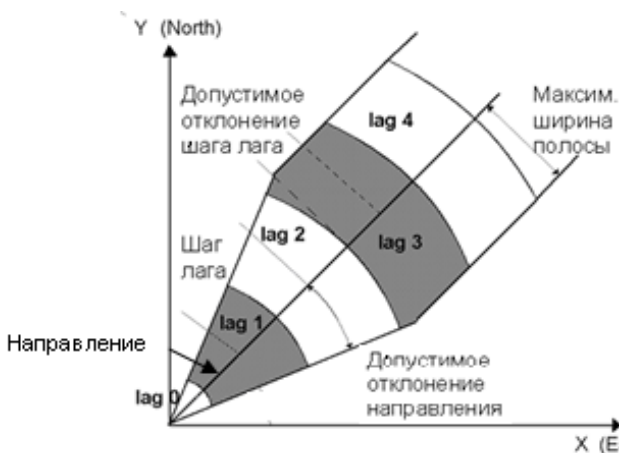
Рис.29. Параметры, задаваемые при вычислении вариограммы по направлению
