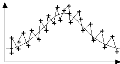
Рис.12. Два примера с постоянной локальной дисперсией
