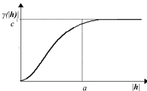
Рис.39. Гауссовая модель
