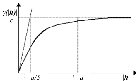
Рис.38. Экспоненциальная модель
