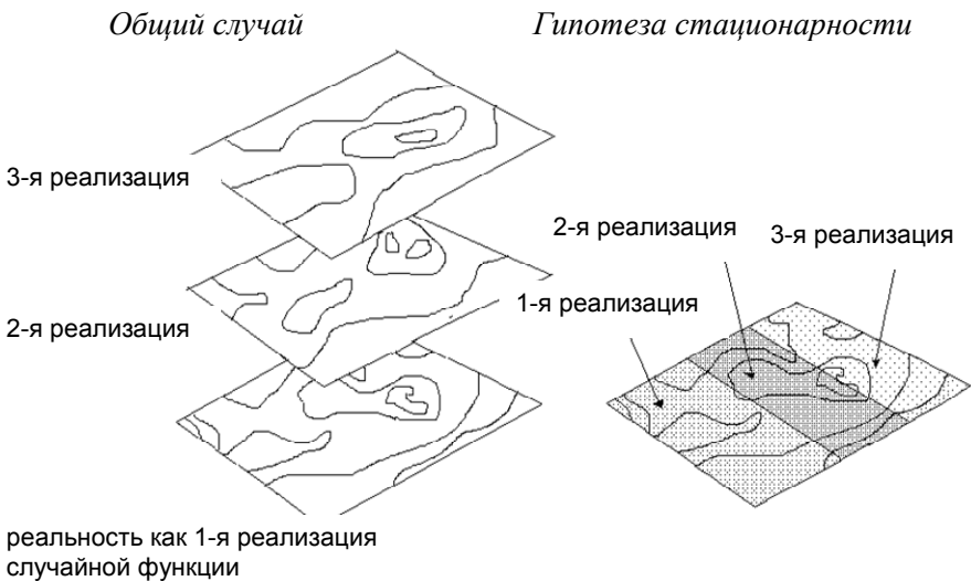
Рис.2. Множество реализаций случайной функции и гипотеза стационарности
