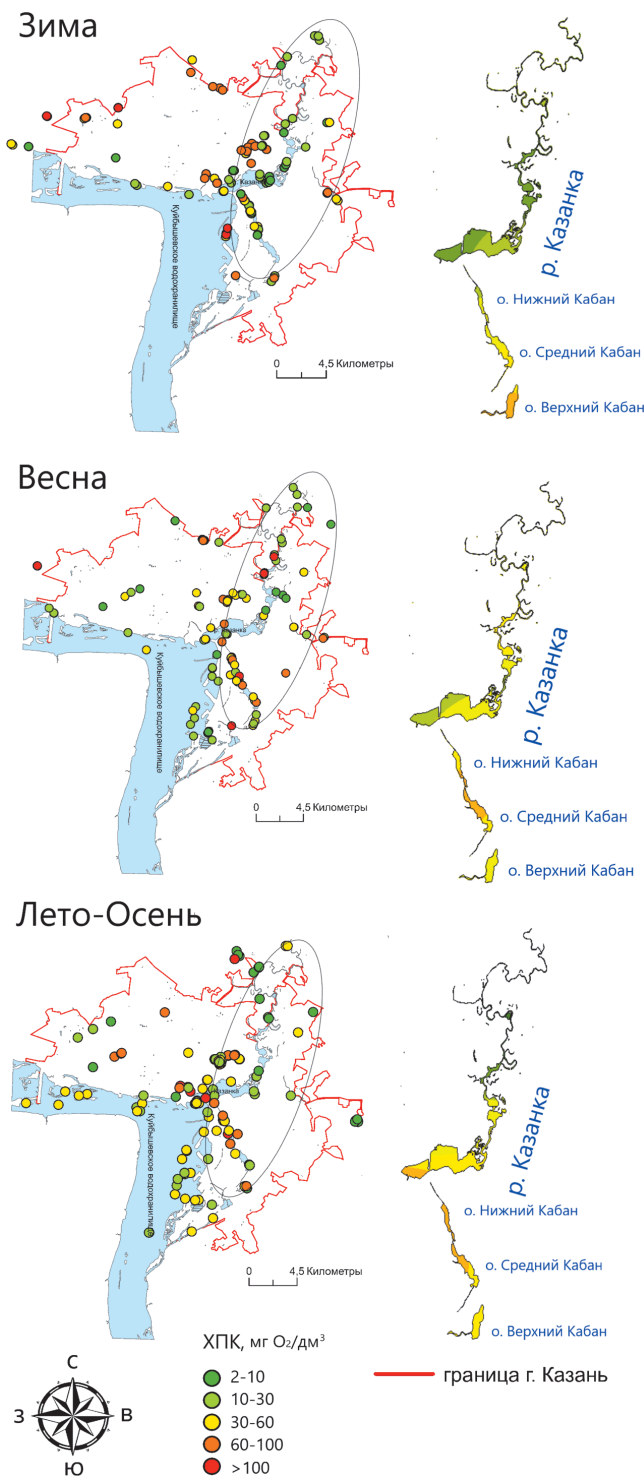
Рис. 2. Распределение ХПК в поверхностных водах. Слева – места отбора гидрохимических проб и значения ХПК справа – распределение ХПК в р. Казанка и оз. Кабан. Примечание: н.о. – не обнаружено
