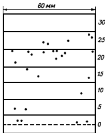
Рисунок 4 - Пример определения среднечасовой ординаты с помощью палетки Савиковского
