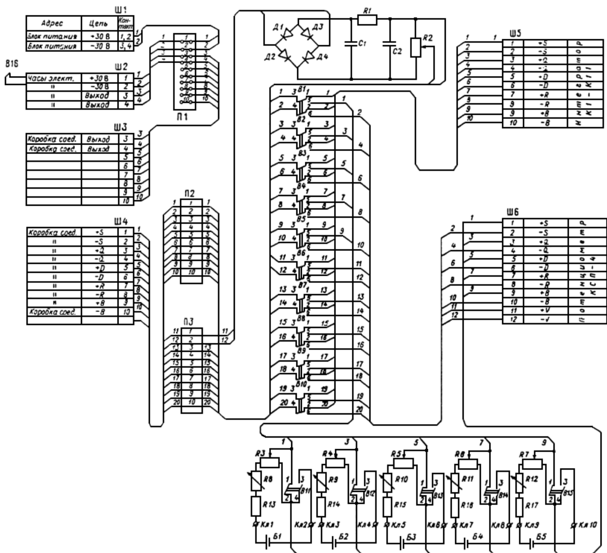
Рисунок Д.9 - Электрическая схема распределительного щита
