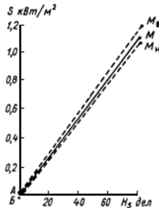
Рисунок 5 - Пример графика зависимости прямой солнечной радиации от ординаты записи сигналов актинометра на диаграммной ленте регистратора
