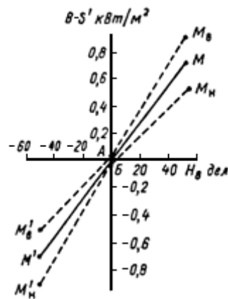
Рисунок 6 - Пример графика зависимости радиационного баланса без прямой солнечной радиации от ординат записи сигналов балансомера на диаграммной ленте регистратора
