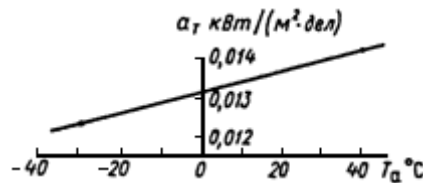
Рисунок В.1 - Зависимость переводного множителя актинометра М-3 N 792 с гальванометром ГСА-1 N 541 от температуры
