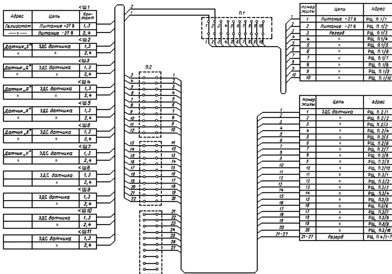
Рисунок Д.16 - Электрическая схема соединительной коробки
