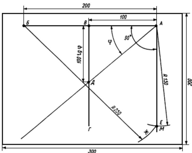
Рисунок Д.15 - Шаблон для контроля установки теневого кольца Корректировку положения теневого кольца производят в следующем порядке.
