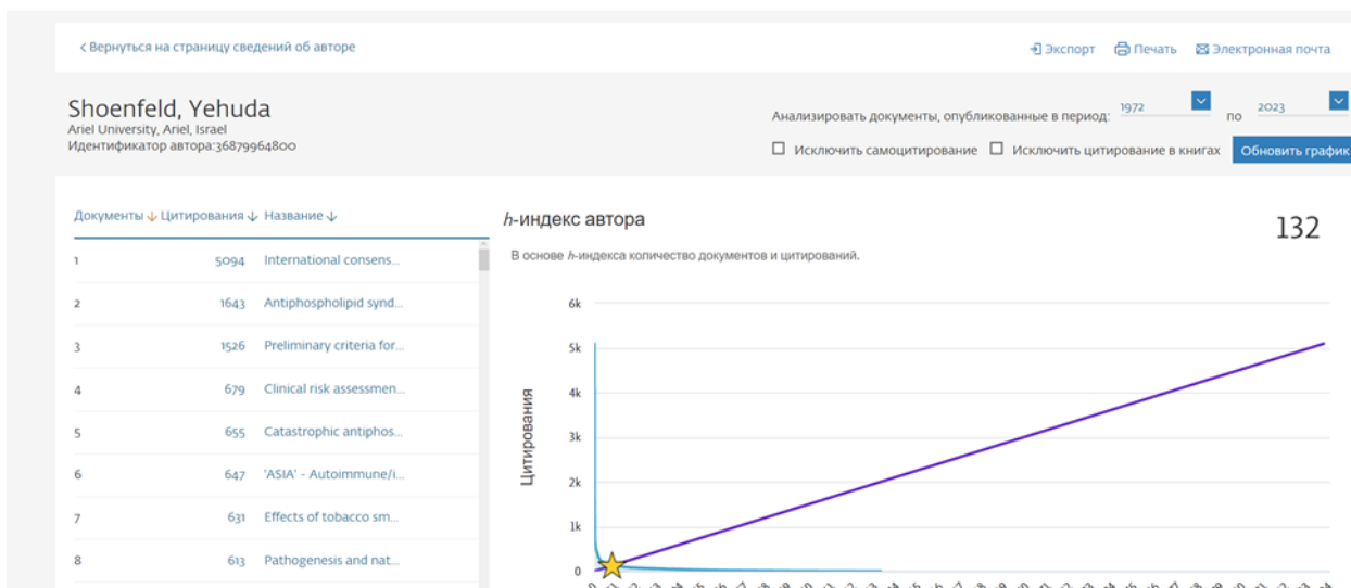
Рис. 20. Значение индекса Хирша для автора Yehuda Shoefeld
