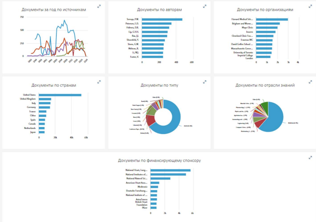
Рис. 11. Результат анализа всех публикаций, найденных по лексеме cardiol* в базе данных Scopus: детализация по годам, источникам, авторам, организациям, странам, типу документов, отрасли знания, финансирующему спонсору
