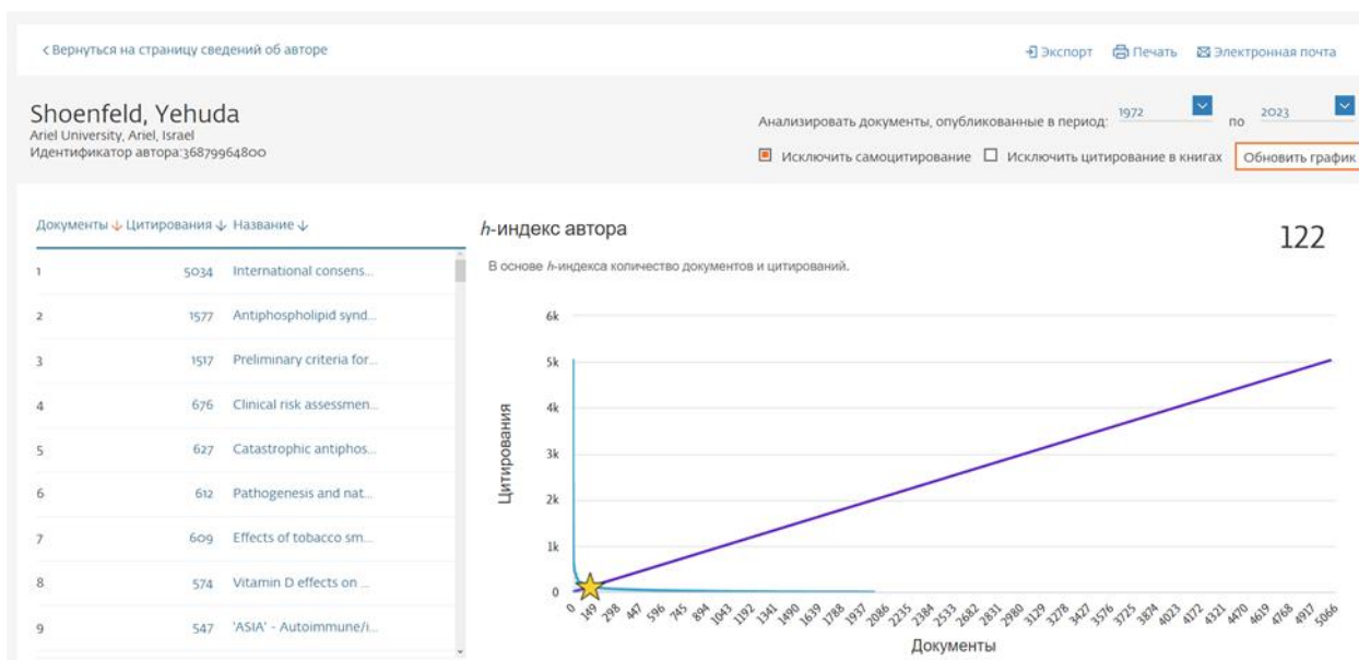
Рис. 21. Вклад самоцитирования в значение индекса Хирша. Из сравнения данных на рис. 20 и 21 видно, что вклад самоцитирования у автора Yehuda Shoefeld не значителен
