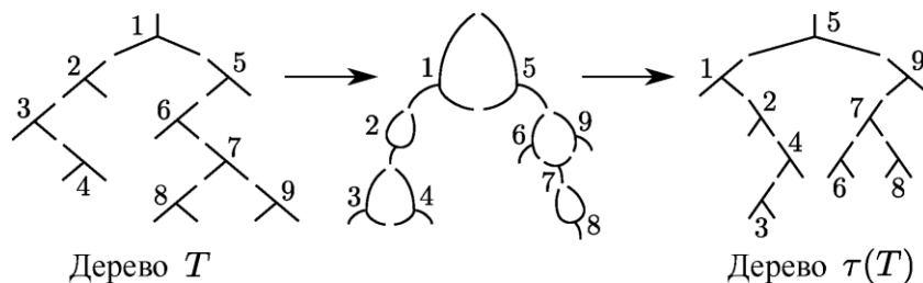
Рис. 1. Преобразование Донахью для дерева, разбитого на триады
