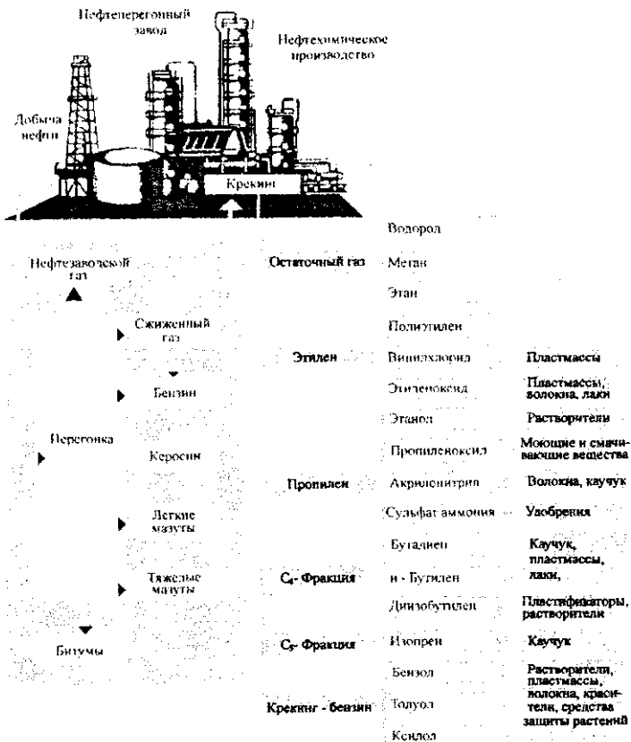
Рис. 6.7. Процесс переработки нефти
