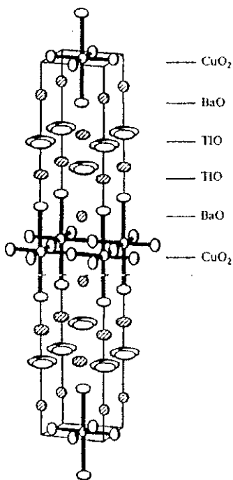
Рис. 6.15. Структура высокотемпературного сверхпроводника
