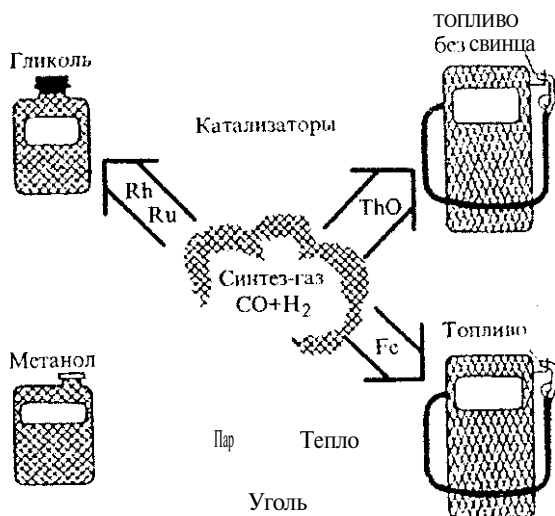
Рис. 6.8. Химические превращения угля
