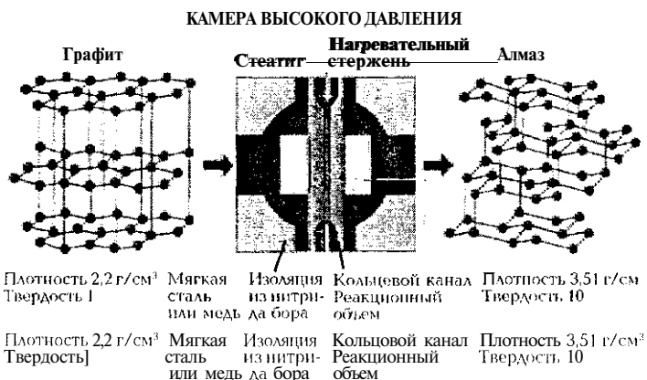
Рис. 6.11. Синтез алмаза
