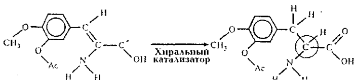
Рис. 6.3. Синтез леводобы
