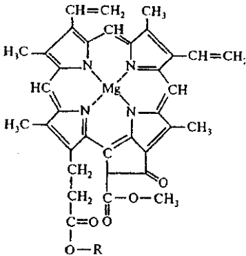
Рис. 7.16. Структура хлорофилла
