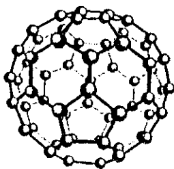
Рис. 6.12. Структура молекулы фуллерена
