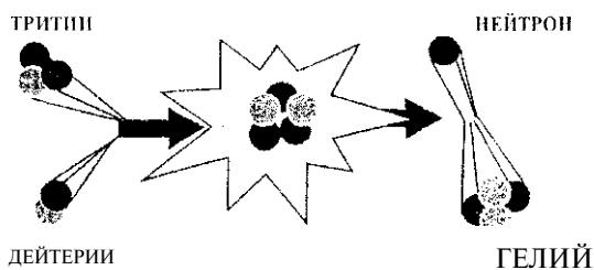
Рис. 4.5. Термоядерный синтез
