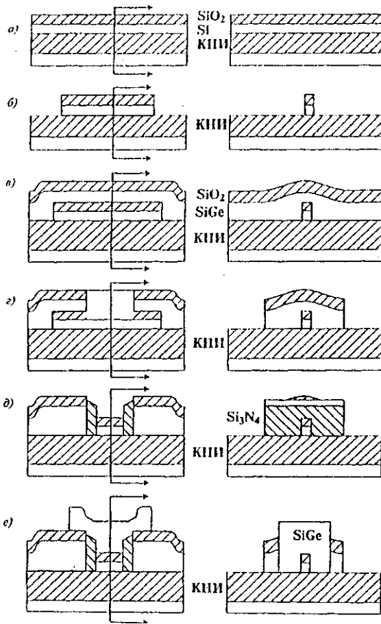
Рис. 8.3. Формирование нанотранзистора
