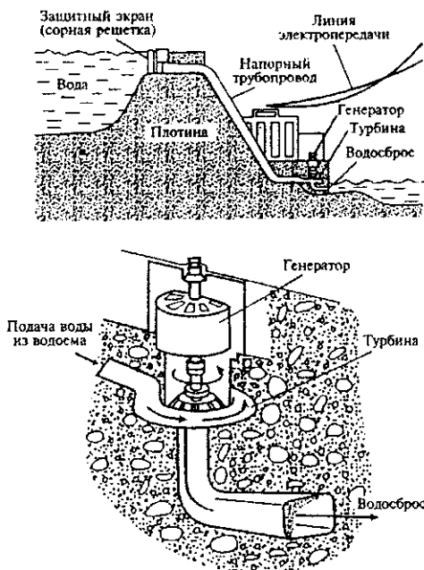
Рис. 9.10. Схема гидроэлектростанции (вверху) и турбогенераторный агрегат (внизу)
