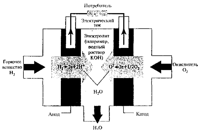
Рис. 9.8. Водород-кислородный топливный элемент
