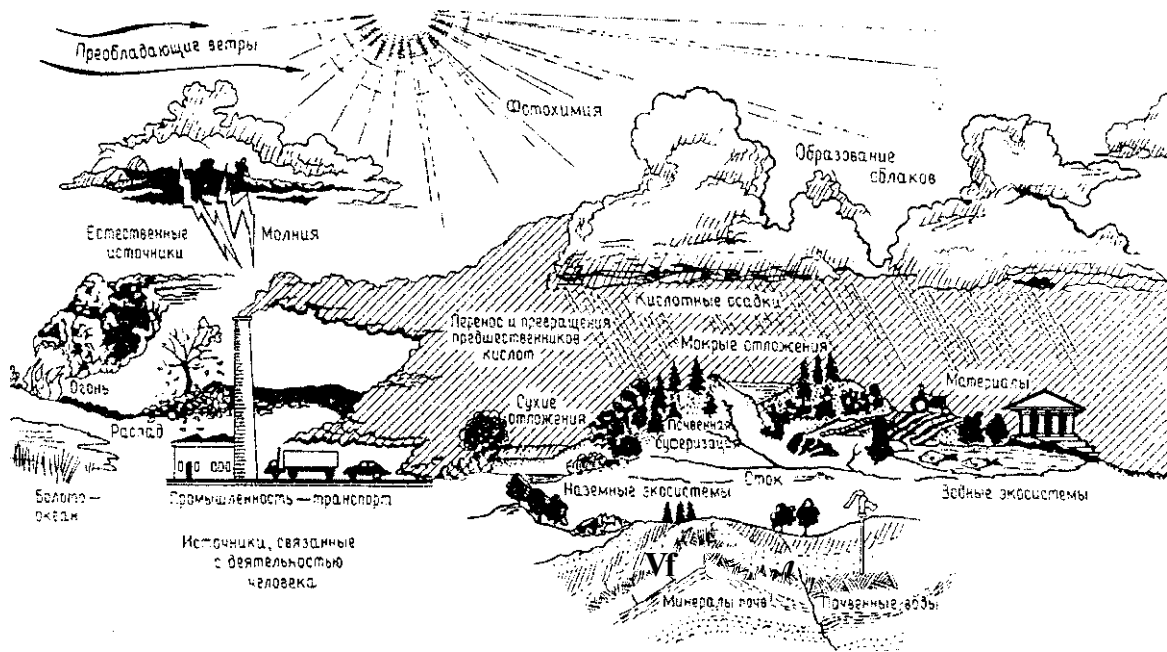
Рис. 10.3. Распространение кислотных осадков
