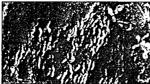
Рис. 6.5. Бактериоподобная структура
