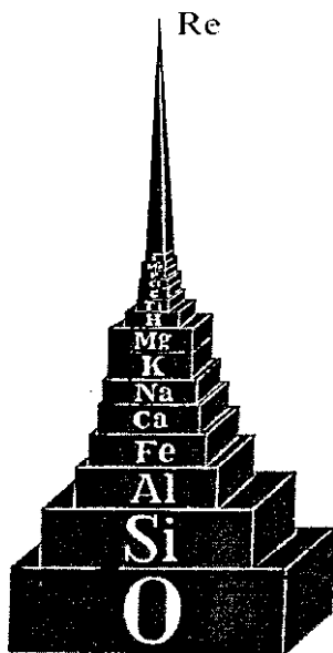
Рис. 6.17. Пирамида распространности химических элементов в земной коре
