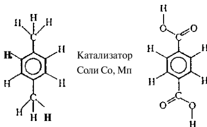
Рис. 6.2. Каталитическое превращение
