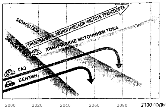
Рис. 9.7. Рост производства автомобилей с разными источниками энергии
