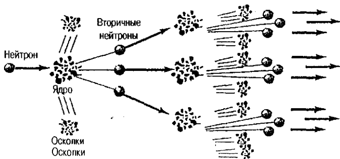
Рис. 4.4. Цепная ядерная реакция
