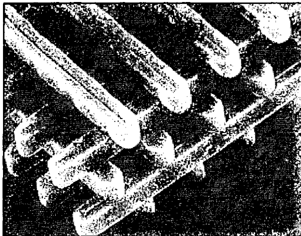
Рис. 8.1. Фотонный кристалл
