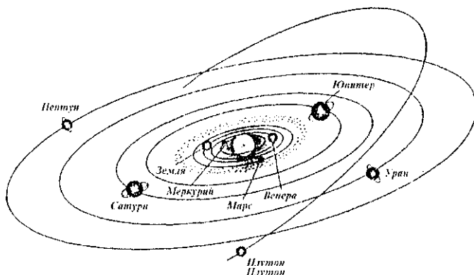
Рис. 5.2. Солнечная система
