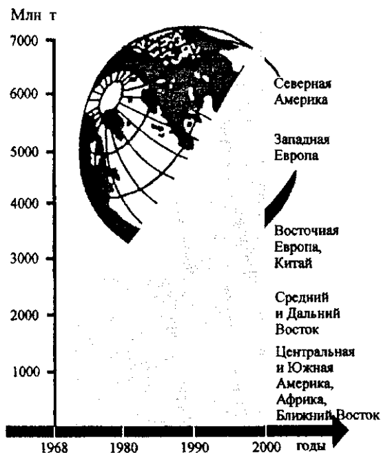
Рис. 6.6. Потребность в нефтепродуктах
