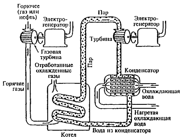
Рис. 9.6. Комбинированный способ получения электроэнергии
