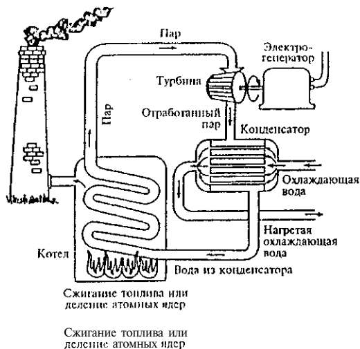
Рис. 9.5. Схема тепловой электростанции
