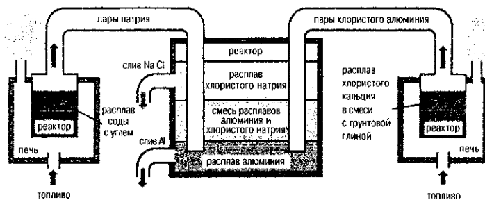
Рис. 9.9. Технология производства алюминия
