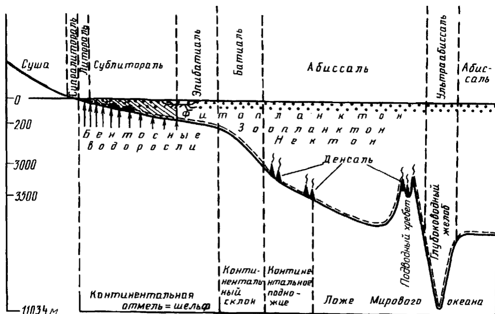
Рис. 1. Биономические зоны: континентальная отмель и шельф: супралитораль – литораль – сублитораль, эпибатталь; континентальный склон: батталь; континентальное подножие, ложе мирового океана: абиссаль – ультраабиссаль
