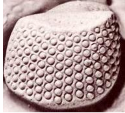
Рис. 16. Шизохроические глаза
