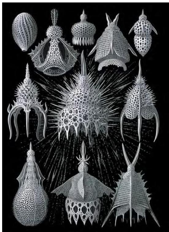
Рис. 14. Скелеты радиолярий
