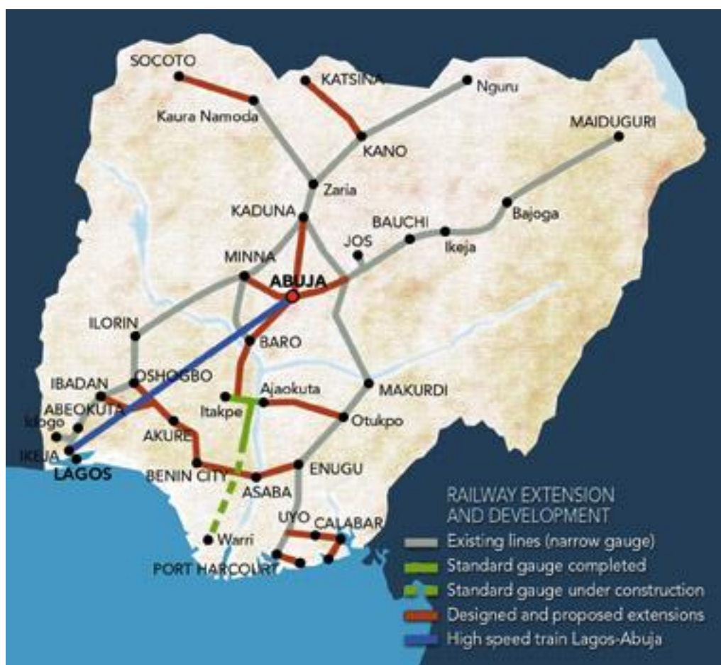
Изображение 1. Схема железнодорожной сети Нигерии. Источник: НЖК
