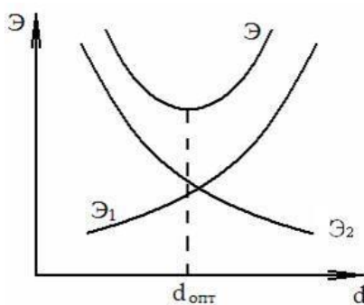
Рис. 4. 5. К определению оптимального диаметра трубопровода
