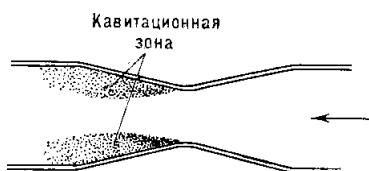
Рис.3. 4. Кавитация
