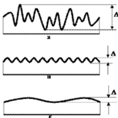
Рис.3. 3. Виды шероховатости:
