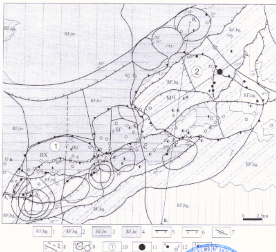
Рис. 2. Структурно-минерогенетическая схема Мало-Чиликетской кварцевой зоны: 1 — бугарихтинская свита, верхняя подсвита; 2 — бугарихтинская свита; 3 — хайвергинская свита; 4 — хорлухтакская свита; 5 — надлиги; 6 — сбросы; 7 — секущая система разломов кинематики; 8 — крутозалегающие сдвиги левой кинематики; 9 — купольно-кольцевые структуры; 10 — купольные; 11 — Верхне-Хайвергинская; 12 — Бугарихтинская; МЧ — Мало-Чиликетская; 1 — мелкие; 10 — рудные узлы; 1 — кварцевые жилы; 2 — жилко-кварцевые; 11 — месторождение Жила 283; 12 — проявления: а — смешанного типа, б — неравномернозернистого метаморфического кварца, в — средне-мелкозернистого гранулоидного кварца, г — гигантозернистого первичнокристаллического кварца
