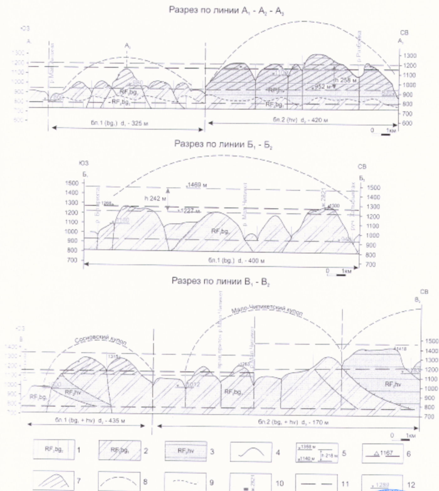
Рис. 4. Профили современной поверхности денудационно-аккумулятивного рельефа с гипсометрическими уровнями рудоносности: 1 — верхний горизонт бугарихтинского комплекса; 2 — нижний горизонт бугарихтинского комплекса; 3 — хайбергский комплекс; 4 — современная поверхность денудационно-аккумулятивного рельефа; 5 — абсолютные отметки вершин, зона выноса кварца и гранулированного кварца; 6 — фоновые абсолютные отметки рудомещающих блоков; 7 — положение предполагаемых зон выноса кварца и гранулированного кварца; 8 — купольные структуры; 9 — предполагаемые линии надвига; 10 — жилы, выходящие на поверхность; 11 — водоносность; 12 — уровень поверхности воды и ее абсолютные отметки
