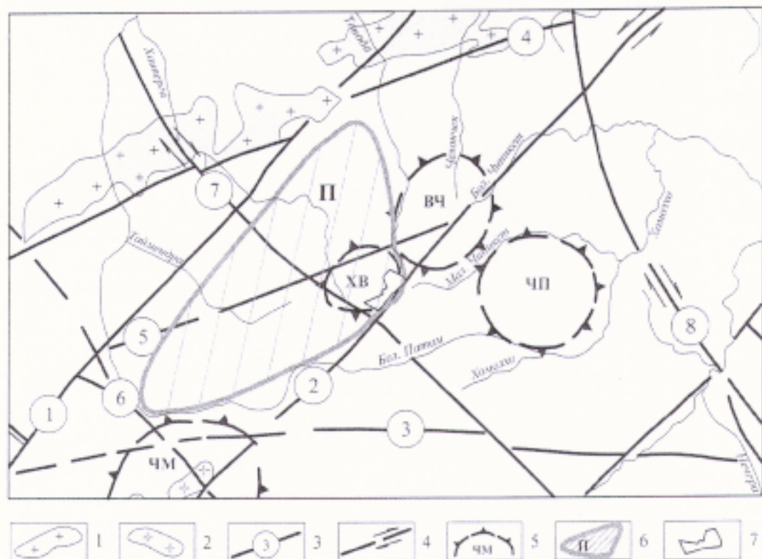
Рис. 1. Положение Патомского кварценосного района в региональной структуре: 1 — гранитоиды верхнего протерозоя; 2 — гранитоиды верхне-среднего протерозоя; 3 — разломы: 1) Чуйский, 2) Мамский, 3) Вацский, 4) Нирундинский, 5) Верхне-Таймендский, 6) Больше-Патомский, 7) Хайвергинский, 8) Нечерский; 4 — сдвиги; 5 — купольные структуры: ЧМ — Чумаркойская, ХВ — Хайвергинская, ВЧ — Верхне-Челонченская, ЧП — Чипикетская; 6 — границы Патомского кварценосного района; 7 — Мало-Чипикетская кварценосная зона
