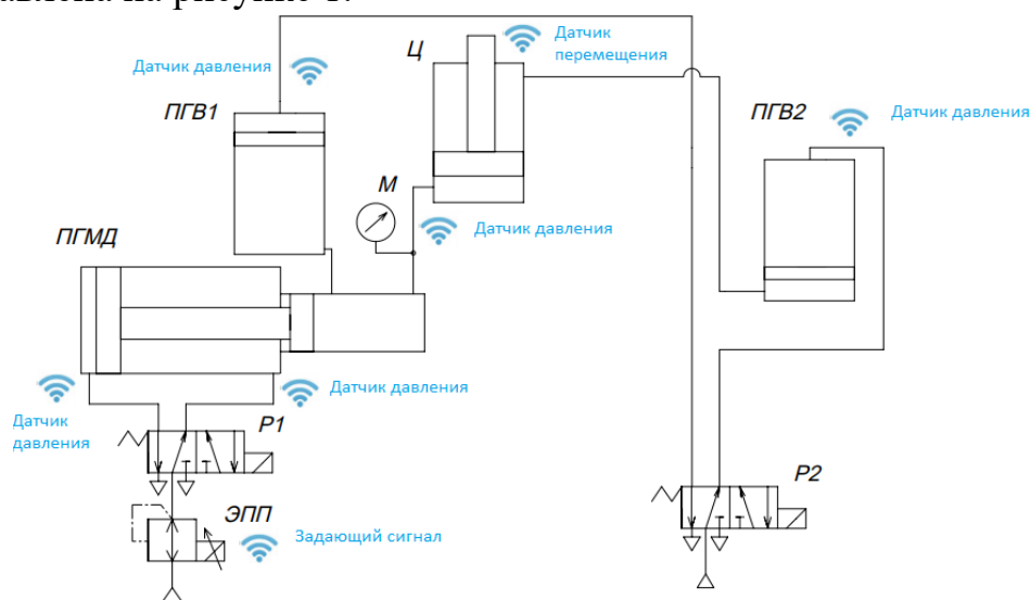
Рисунок 1 - Схема пневмогидравлического привода с возможностью удаленной диспетчеризации
