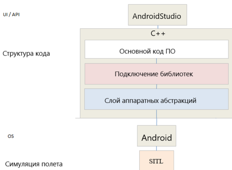
Рис. 1 – Архитектура приложения.
