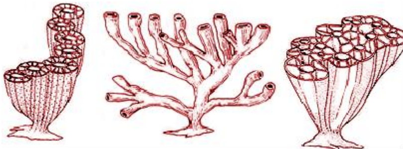
Рис. 37. Колониальные археоциаты
