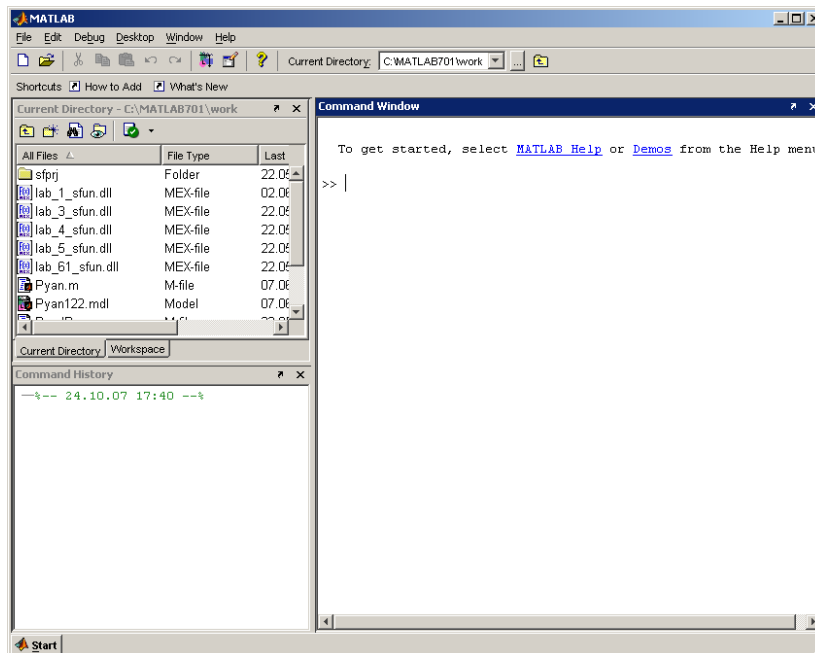
Рис. 1. Окно MATLAB
