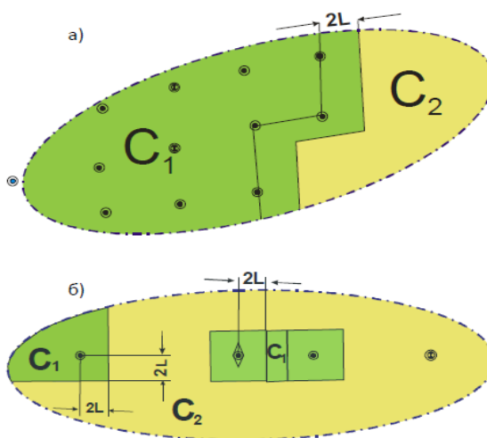
Рисунок 6.7 Выделение запасов категории C_1 и C_2 на разведываемых залежах
