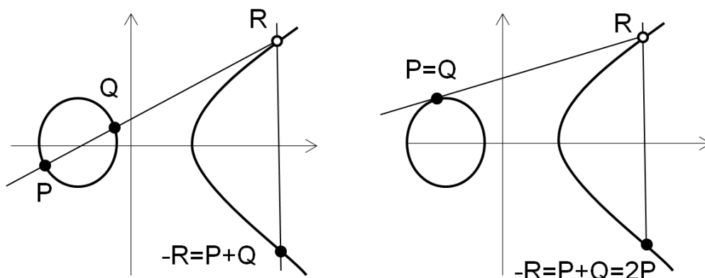
Рис. 6.2.1. Эллиптические кривые
