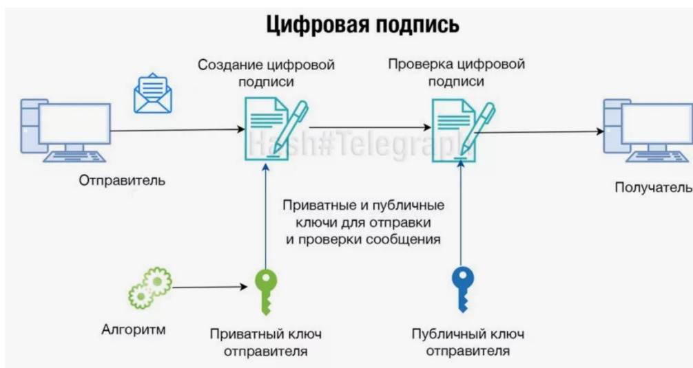
Рис. 4.4.1. Наложение цифровой подписи на документ
