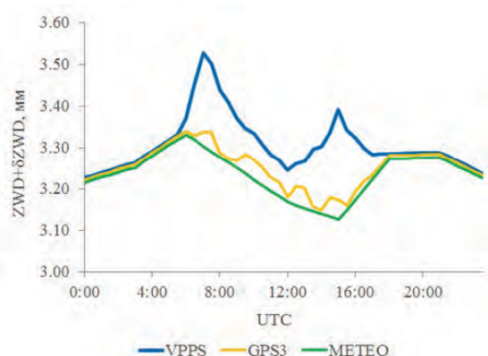
Рис. 1. Средний суточный ход фоновых значений ZWD в приземном слое в июле по данным метеостанции (METEO); Суммарный суточный ход ZWD и \delta ZWD на базовой станции (GPS3) и станции мониторинга (VPPS)
