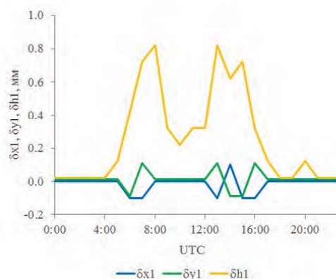
Рис. 2. Ошибки координат станции мониторинга VPPS, вносимые локальными неоднородностями, представленные топоцентрической системе отсчета
